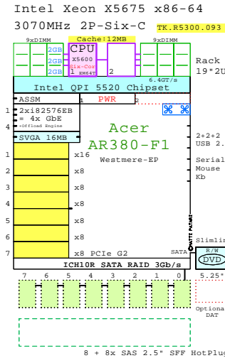
Acer AR380-F1 x86-64 2U
